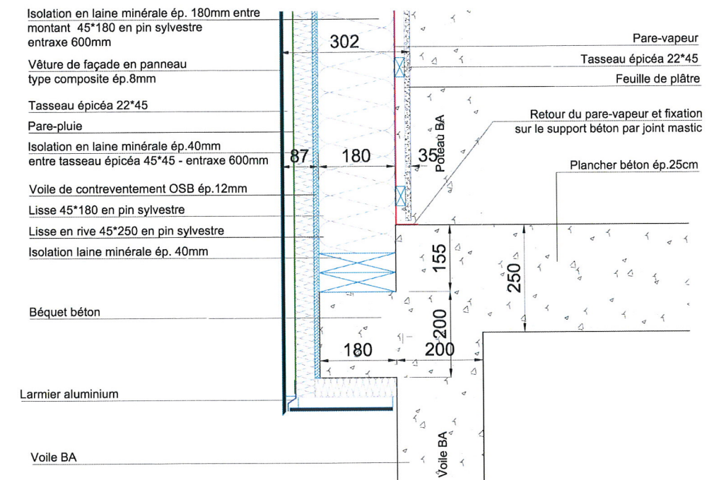
Détail 3 soubassement
