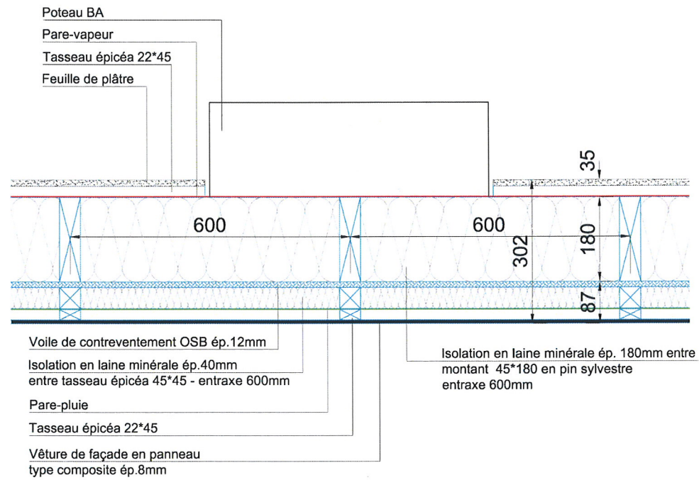
Détail 2 plancher
